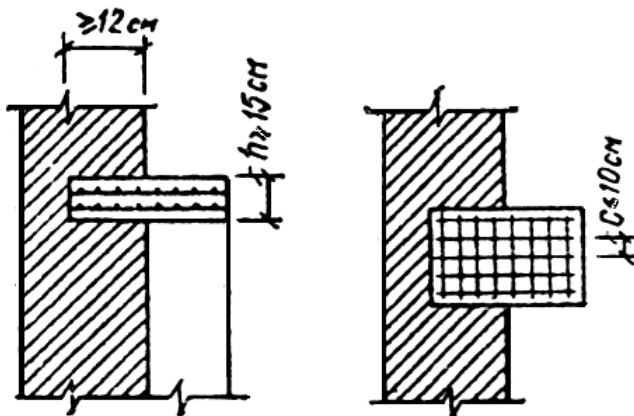
Рис. 13. Железобетонные распределительные плиты
