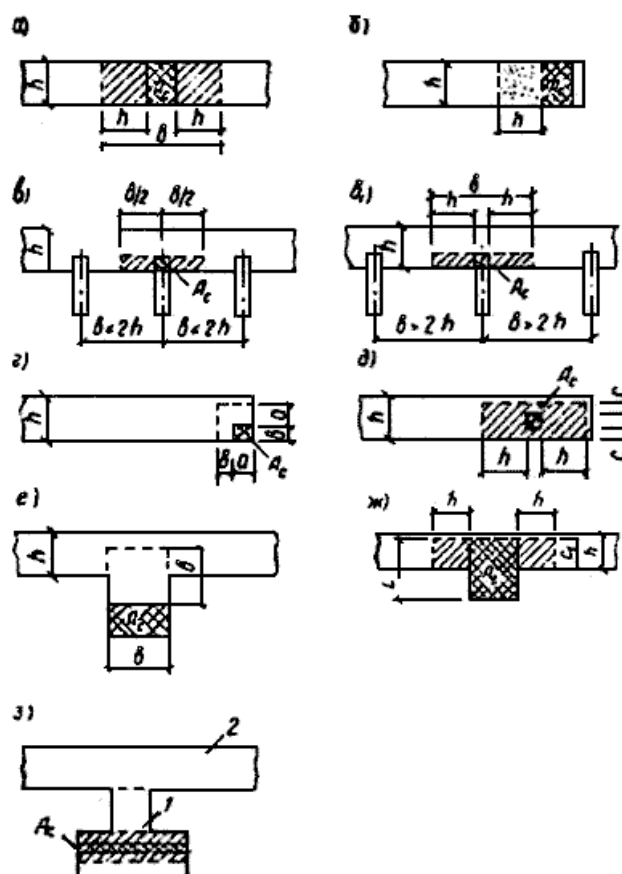
Рис. 9. Определение расчетных площадей сечений при местном сжатии а — з — различные случаи местного сжатия
