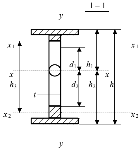
Рис. 23. Схема участка балки с перфорированной стенкой
