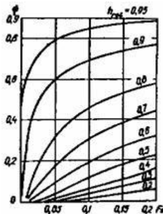
Рис.35. Графики значений коэффициента y
