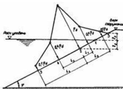
Рис.11. Эюра максимального расчетного волнового давления на откос, укрепленный плитами
