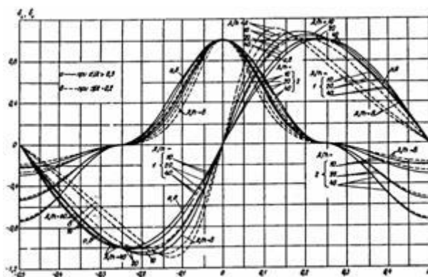
Рис 15. Графики значений коэффициентов сочетания инерционного d_i (графики 1) и скоростные d_v , (графики 3) компонентов силы от воздействия волн
