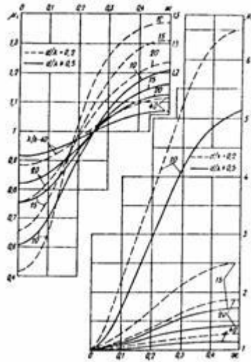
Рис.22. Графики значений инерционного m_i , и скоростного m_v коэффициентов фазы
