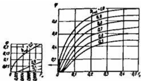
Рис. 36. Графики значений коэффициента j
