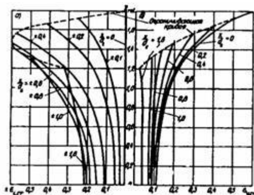
Рис.25. Графики значений инерционного e_{i,cr} и скоростного e_{v,cr} коэффициентов
