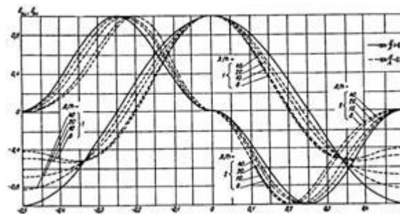
Рис.23. Графики значений коэффициентов сочетания d_{zi} инерционного (графики 1) и d_{zv} - скоростного (графики 2) компонентов вертикальной линейной нагрузки от волн
