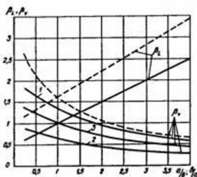
Рис.17. Графики значений инерционного b_i и скоростного коэффициентов формы (для эллиптических преград - сплошные линии, при призматических - штриховые линии) в зависимости от a/b (для Q , q и P_x ) или b/a (для P_z )
