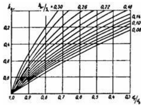
Рис. 2. Графики значения коэффициента kbr
