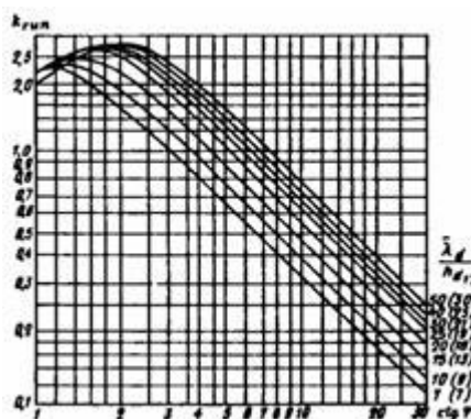
Рис. 10*. Графики значений коэффициента k_{grun}
