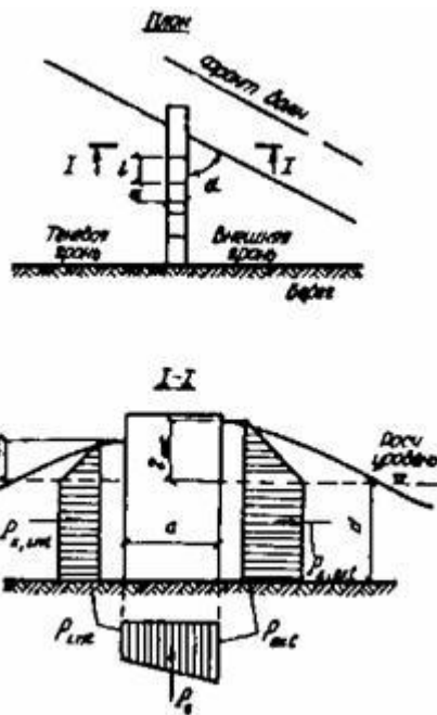
Рис. 30. Эпюры волнового давления на буну
