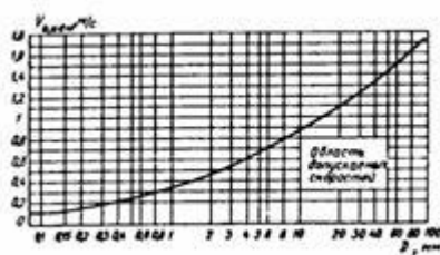
Рис.7. График допустимых значений неразмывающих донных скоростей
