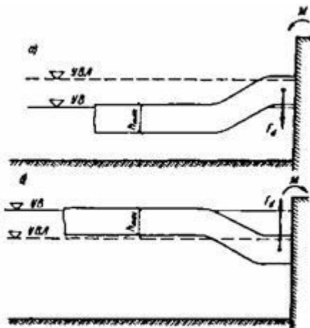
Рис. 37*. Схемы к определению нагрузок от примерзшего к сооружению ледяного покрова при изменении уровня воды (УВ)
