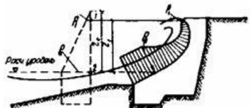
Рис.29. Эпюра давления воли на криволинейный участок волнозащитной стены
