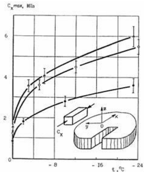
Рис.2. Зависимость максимального предела прочности пресноводного льда при одноосном сжатии от температуры.
