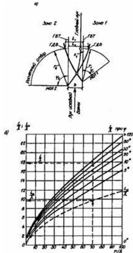
Рис. 9. Схема (а) и графики (б) для определения величин \beta_i и l_{\alpha}
