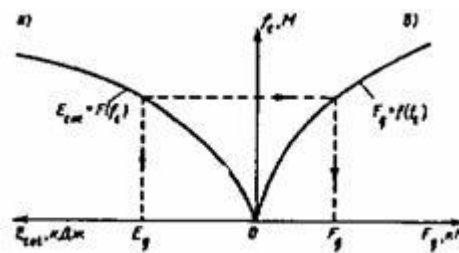
Рис. 33. Схема построения графиков зависимости деформаций отбойного устройства (и причального сооружения) f_t а - от энергии E_{tot} ; б - от нагрузки F_q
