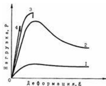
Рис.1. Диаграммы "нагрузка - деформация" для льда, испытываемого при различных постоянных скоростях деформации: \dot{\epsilon}_1 < \dot{\epsilon}_2 < \dot{\epsilon}_3 < \dot{\epsilon}_4 . 1, 2 - пластическое разрушение; 3 - хрупко - пластическое разрушение; 4 - хрупкое разрушение.
