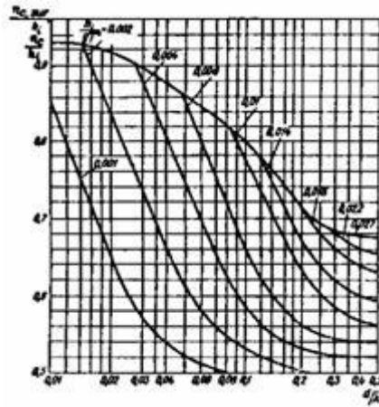
Рис. 3. Графики для определения значений h_c/h_i в мелководной и h_c, \text{surf}/h_i в прибойной зонах
