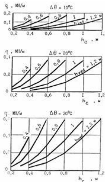
Рис.40. График значений нагрузки q
