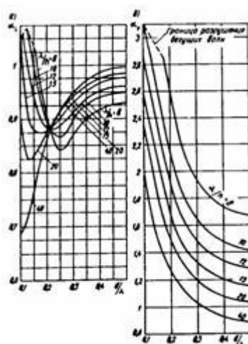
Рис.16. Графики значений инерционного a_i и скоростного a_v коэффициентов глубины
