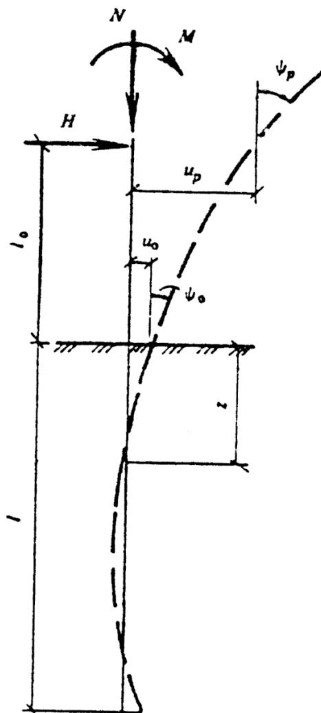
Схема нагрузок на сваю
