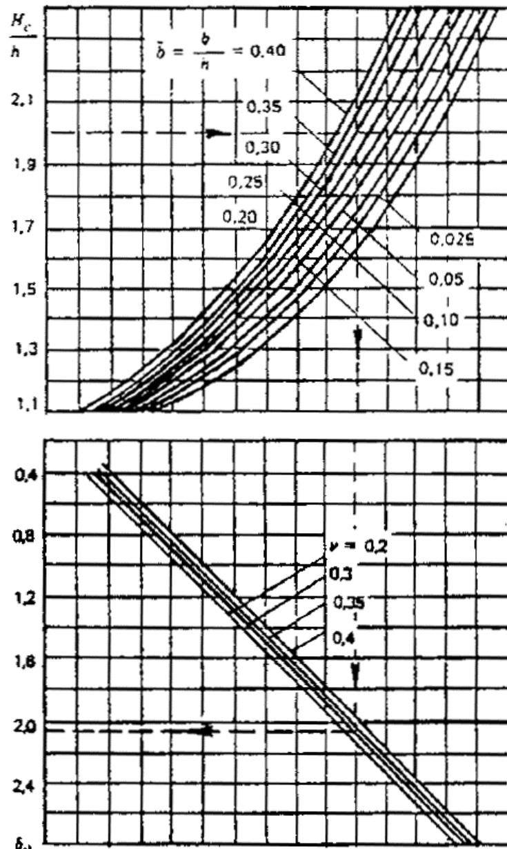
Номограмма для определения значений \delta_0
