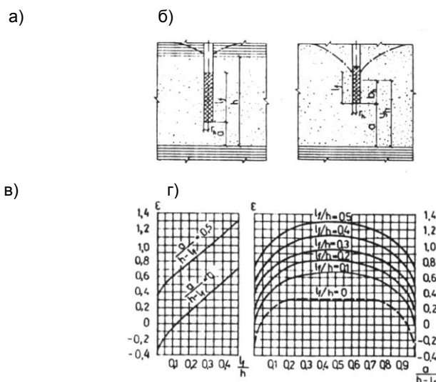
Черт. 3 К расчету сопротивления скважин на гидрологическое несовершенство
