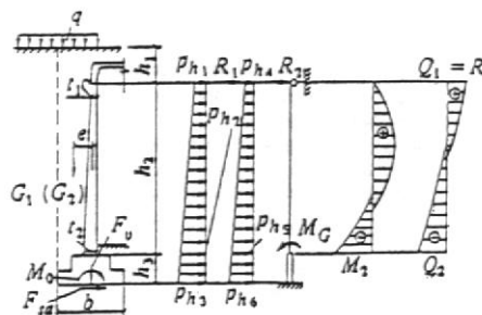
Черт. 3. Расчетная схема стены подвала
