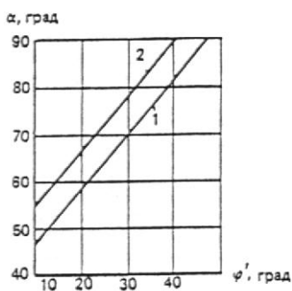
Черт. 6. Графики для определения угла наклона стенок бункеров для связных материалов
