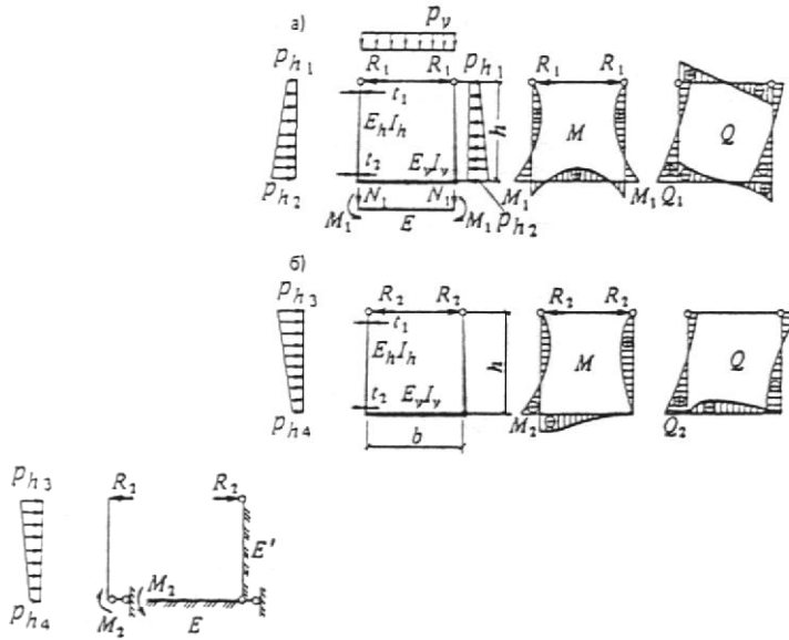
Черт. 4. Расчетная схема тоннеля с шарнирами в уровне плит перекрытия
