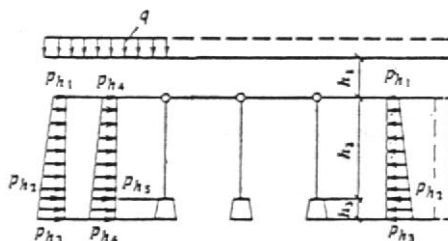
Черт. 2. Расчетная схема поперечной рамы подвала
