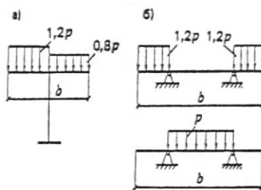
Черт. 7. Распределение интенсивности вертикальной нагрузки на траверсы отдельно стоящих опор и эстакад
