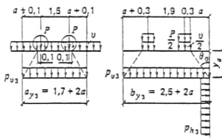
Черт. 4. Схема давления от автомобильной нагрузки АК при
